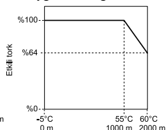
Ortam hava sıcaklığı ve rakım
