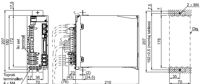
Montaj deliği diyagramı
