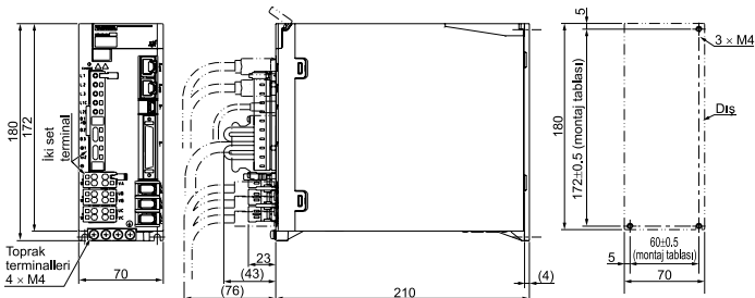
Montaj deliği diyagramı
